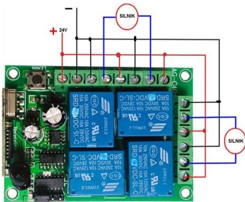
Przykładowe podłączenie silników 24V do sterownika Praca lewo/prawo +24V
